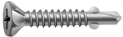
PARAF. CABEÇA CHATA DENTADA E PONTA BROCA COM ASAS
